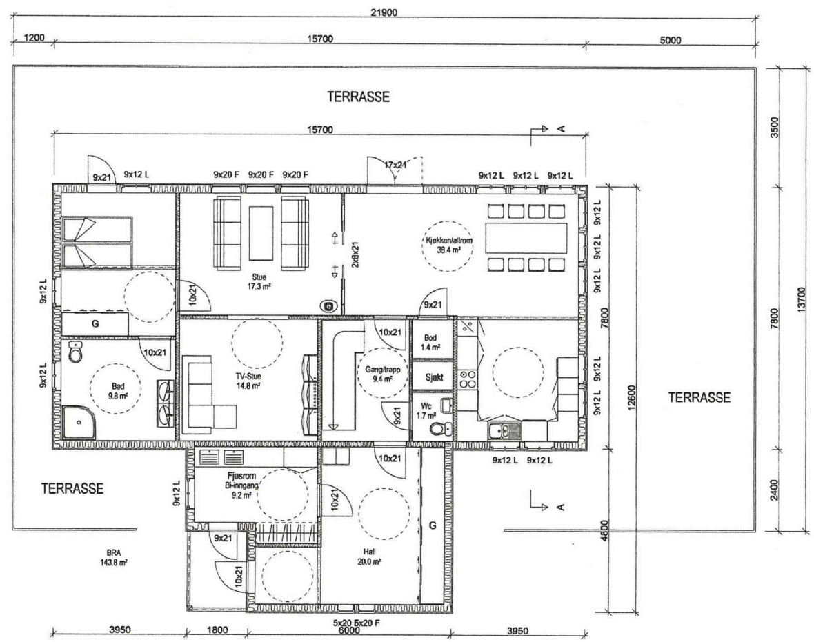
Hovedplan
