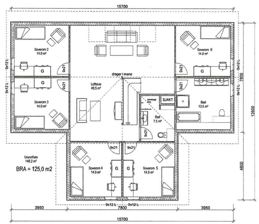
LOFTSPLAN
