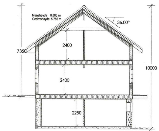
SNITT
