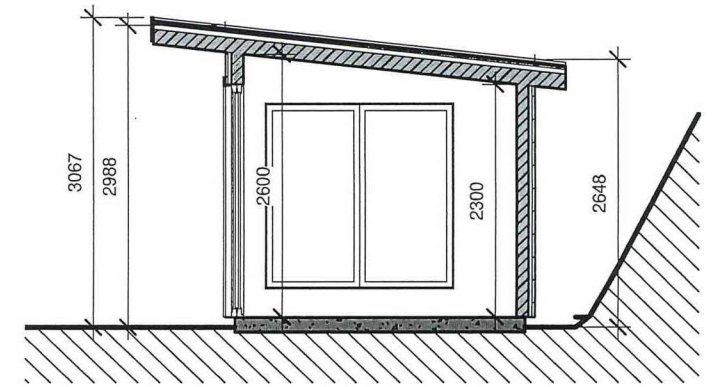
2 Snitt 1 : 50
