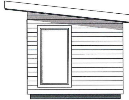
2 Nordøst 1 : 50
