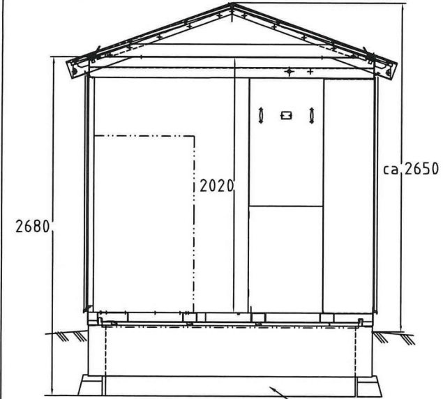
Snitt C-C Oljeoppsamlingskar
