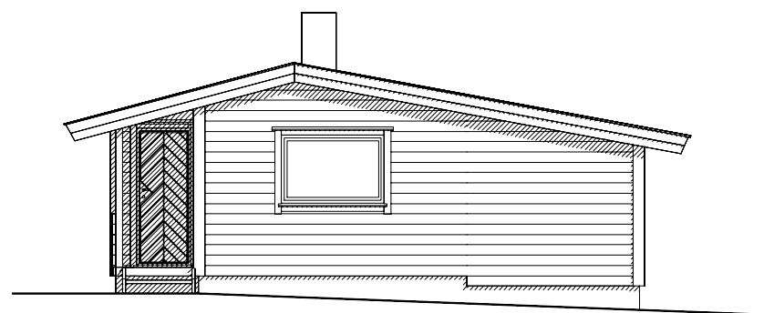
FASADE SØRØST
