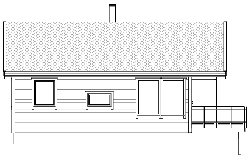
FASADE 1 1 : 100
