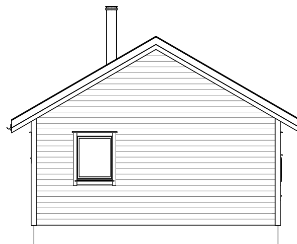
FASADE 4 1 : 100
