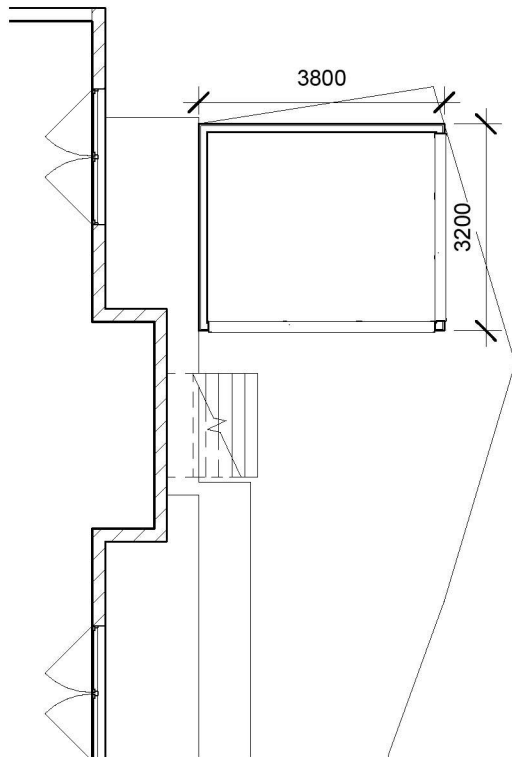
1 Plan 1 : 100
