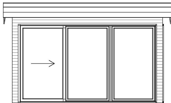
3 Fasade nord 1 : 50
