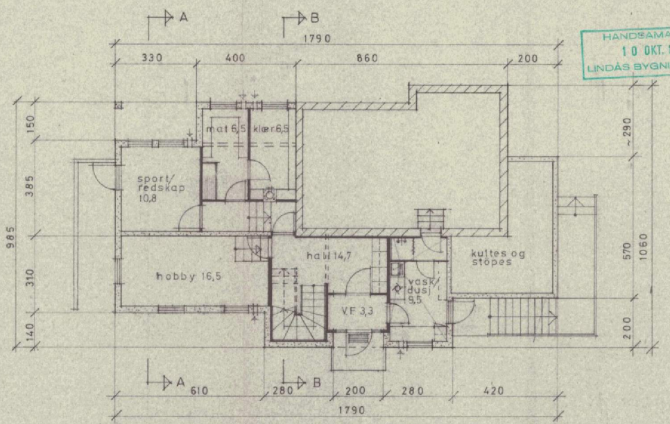
PLAN UNDERETASJE
