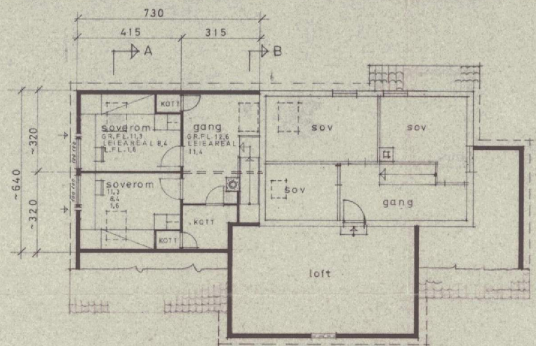
LOFTSPLAN
