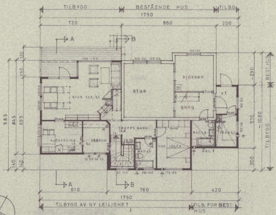
PLAN 1. ETASJE
