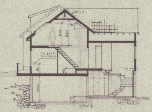
SNITT B-B
