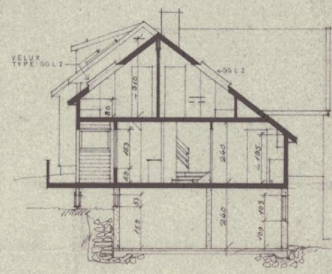
SNITT A-A
