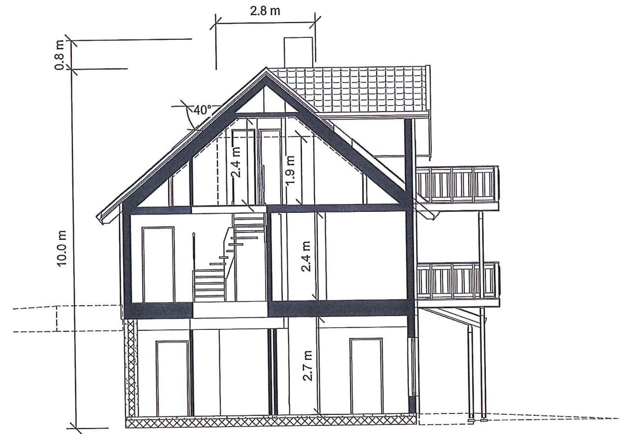
SNITT A-A
