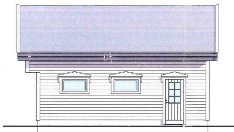
2 Fasade mot sør 1 : 100
