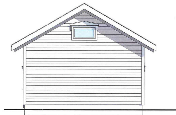
3 Fasade mot øst 1 : 100
