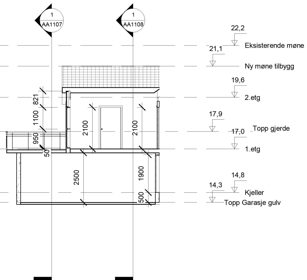
2 Snitt 2 1 : 100
