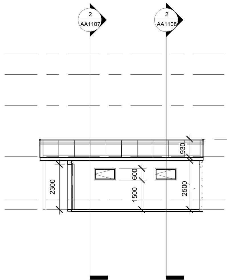
1 Snitt 1 1 : 100
