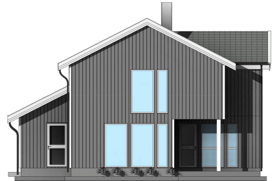
Fasade Vest 1 : 100
