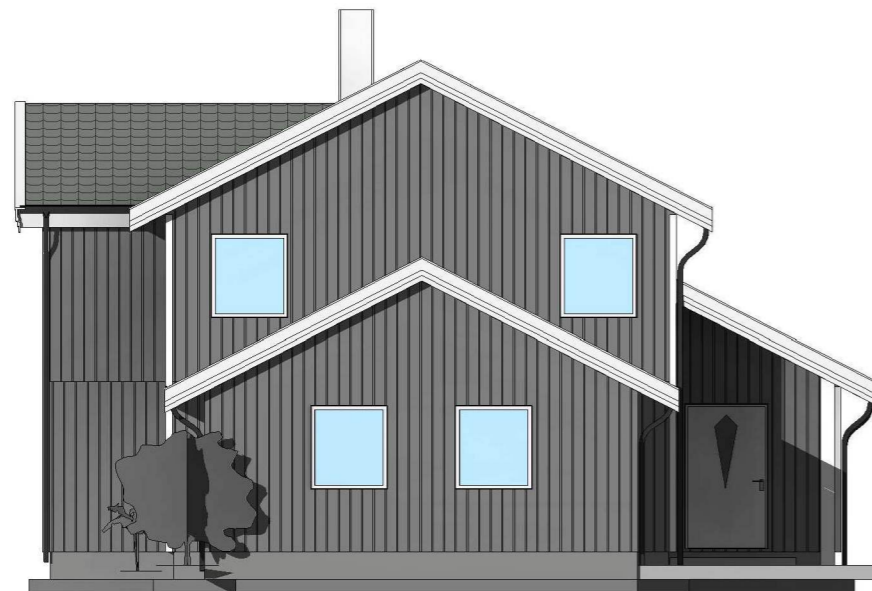
Fasade Øst 1 : 100
