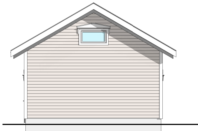
3 Fasade mot øst 1 : 100
