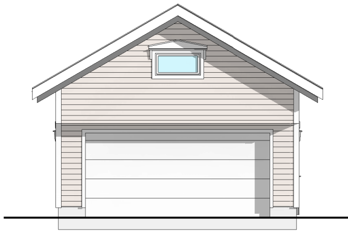
1 Fasade mot vest 1 : 100
