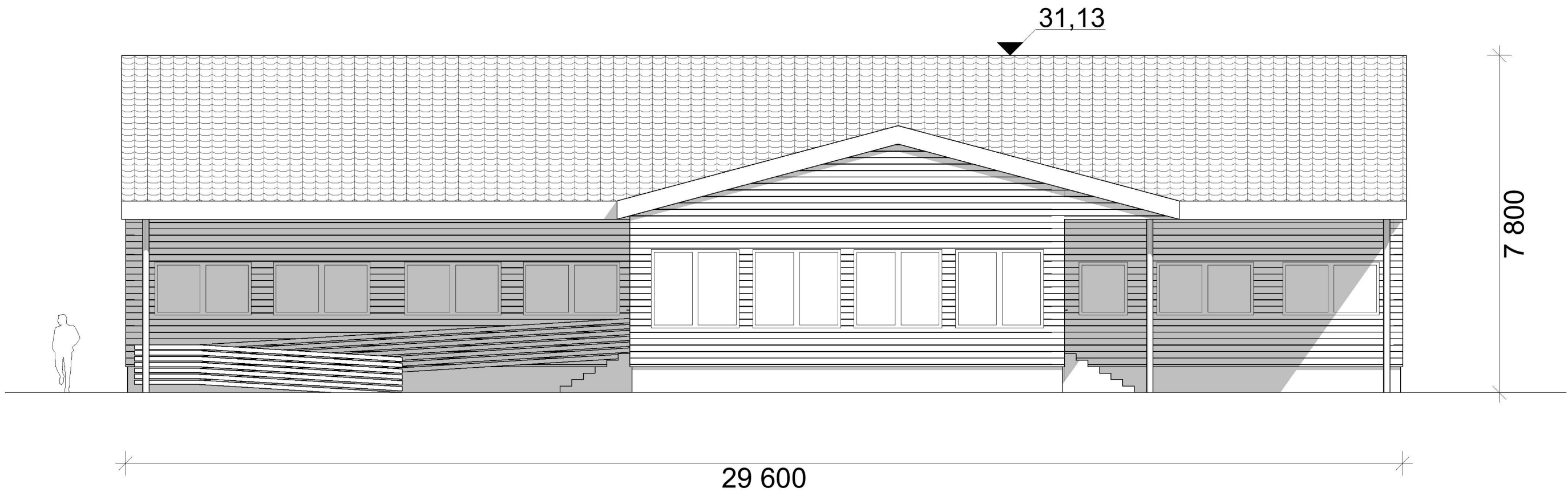
Fasade mot nordøst
