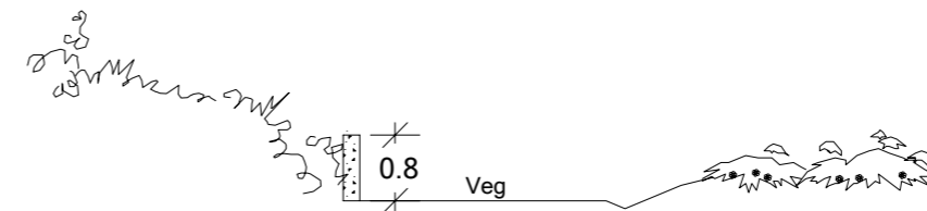
Snitt av mur
