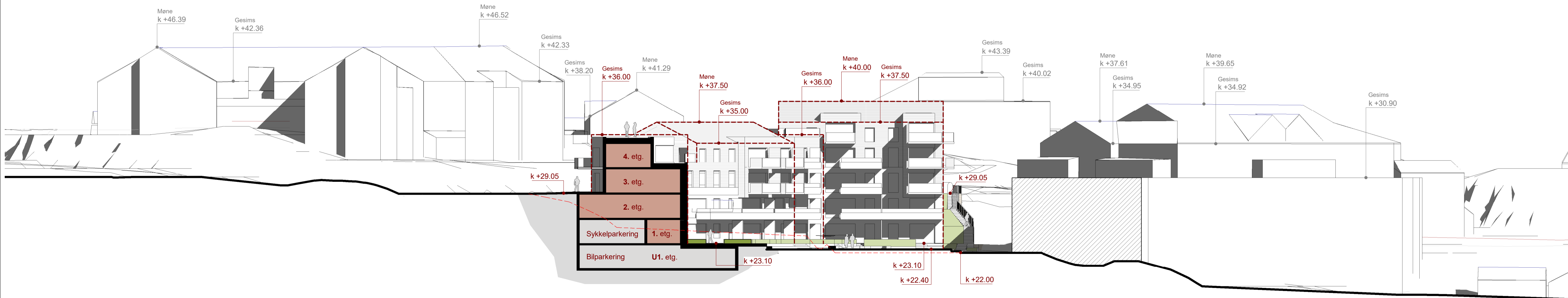
Snitt 2-2 1 : 250
