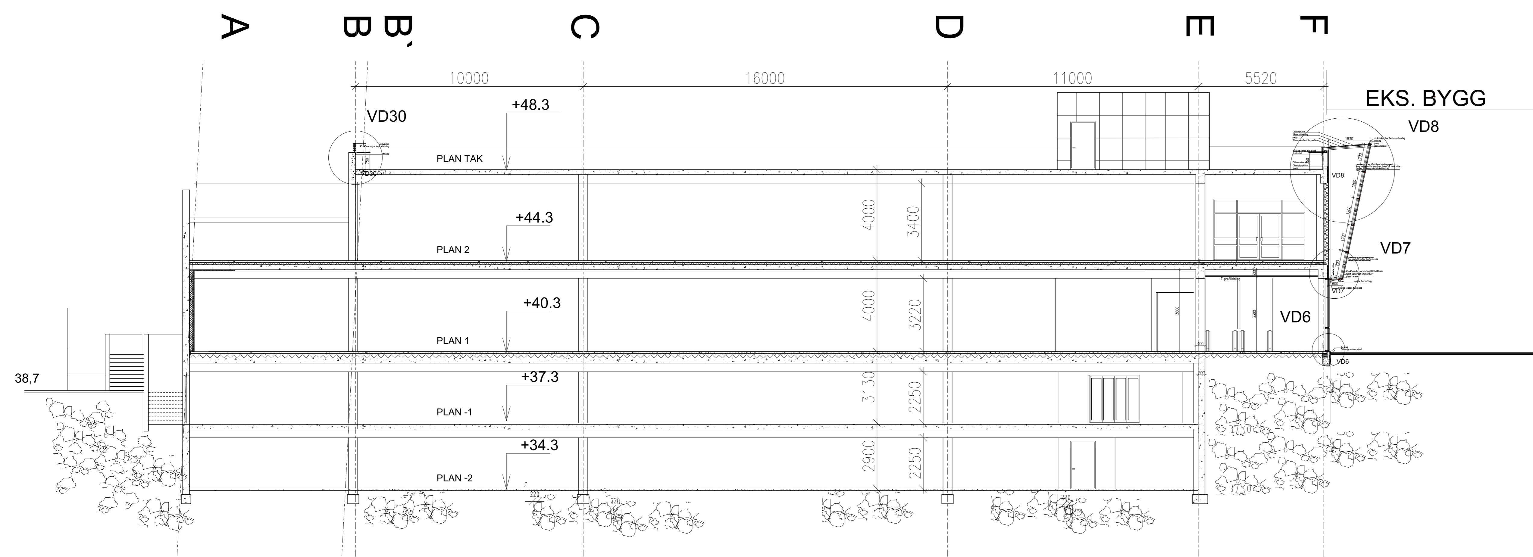
SNITT B-B
