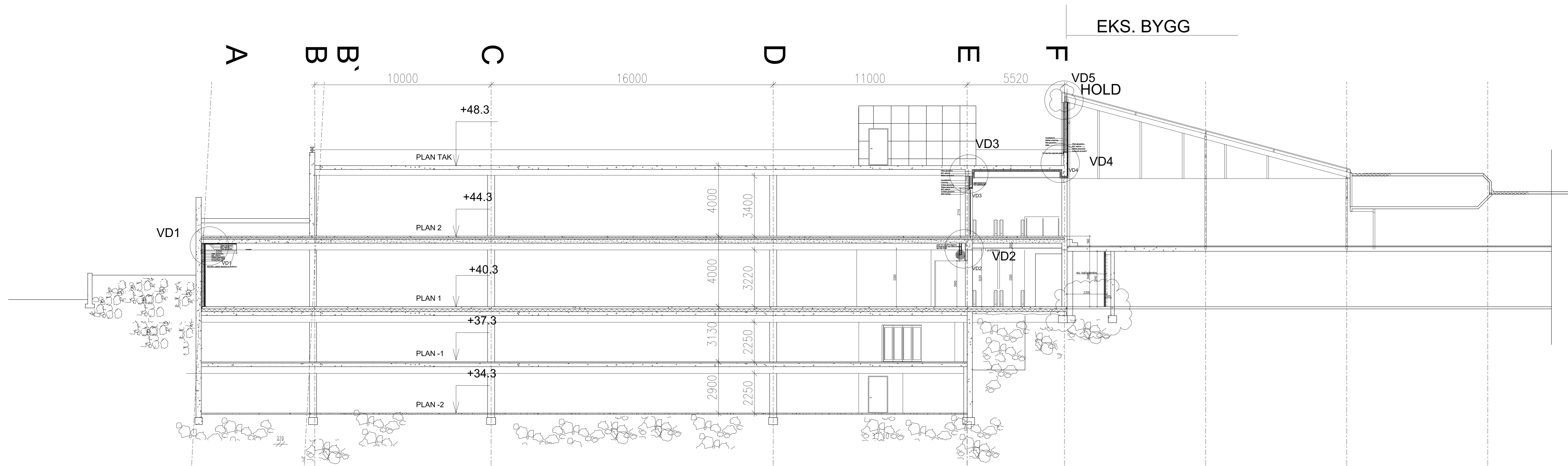
SNITT A-A
