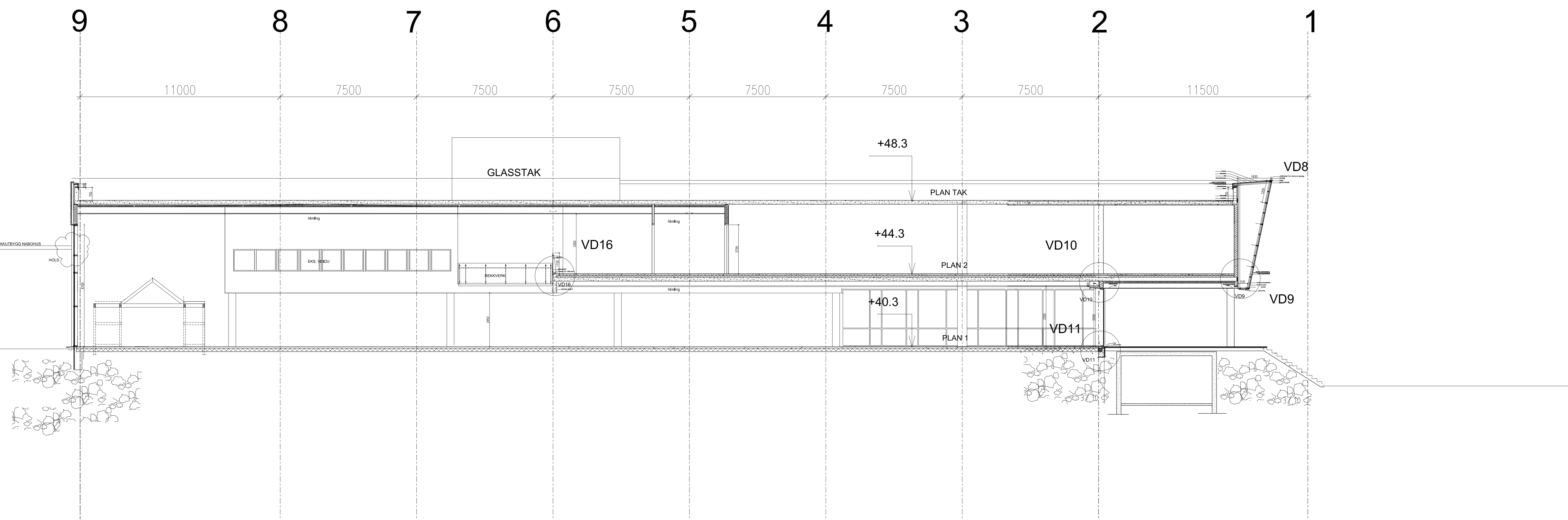
SNITT D-D
