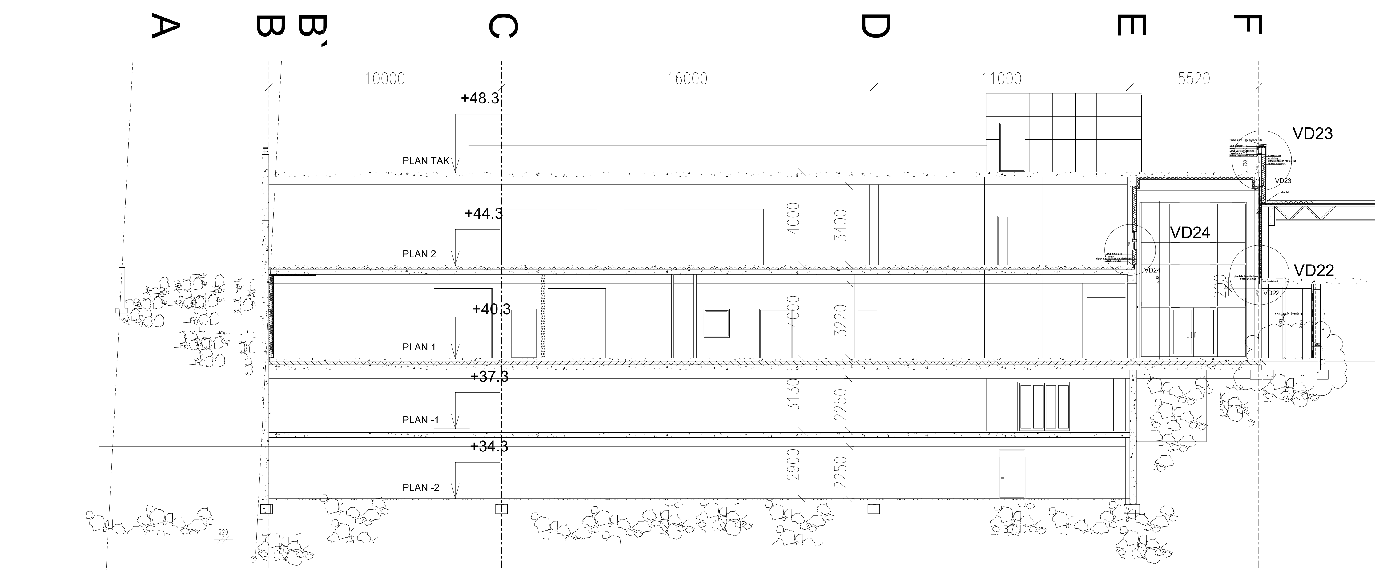
SNITT E-E
