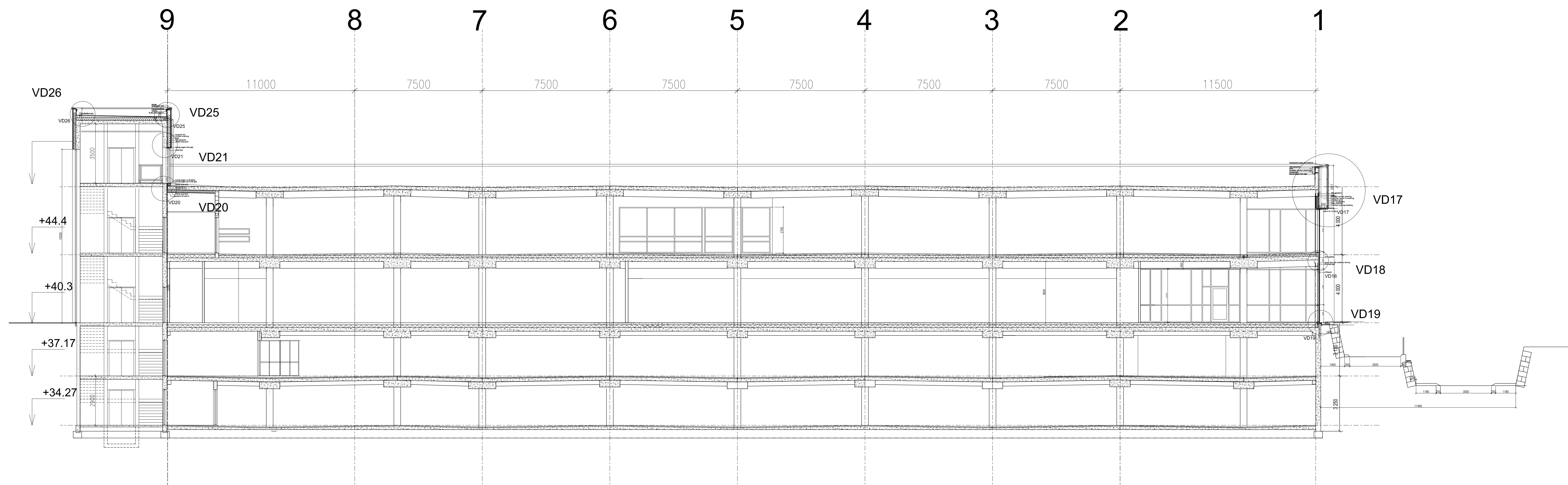
SNITT F-F
