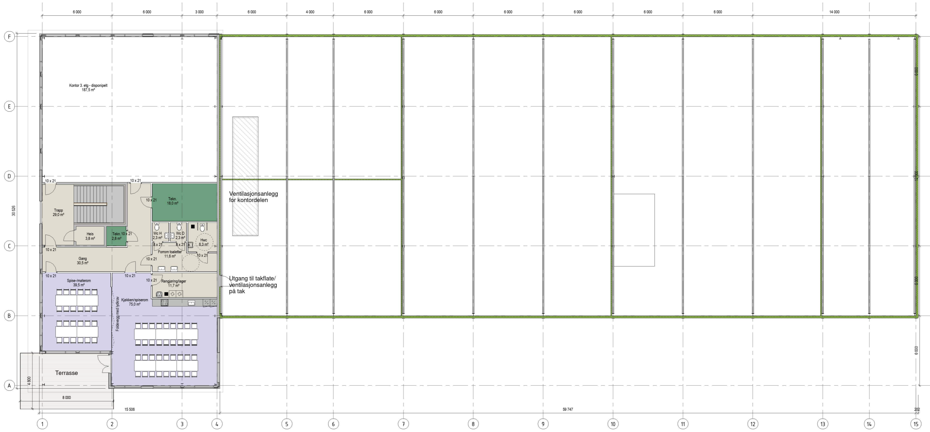
300 Plan 3 1 : 100
