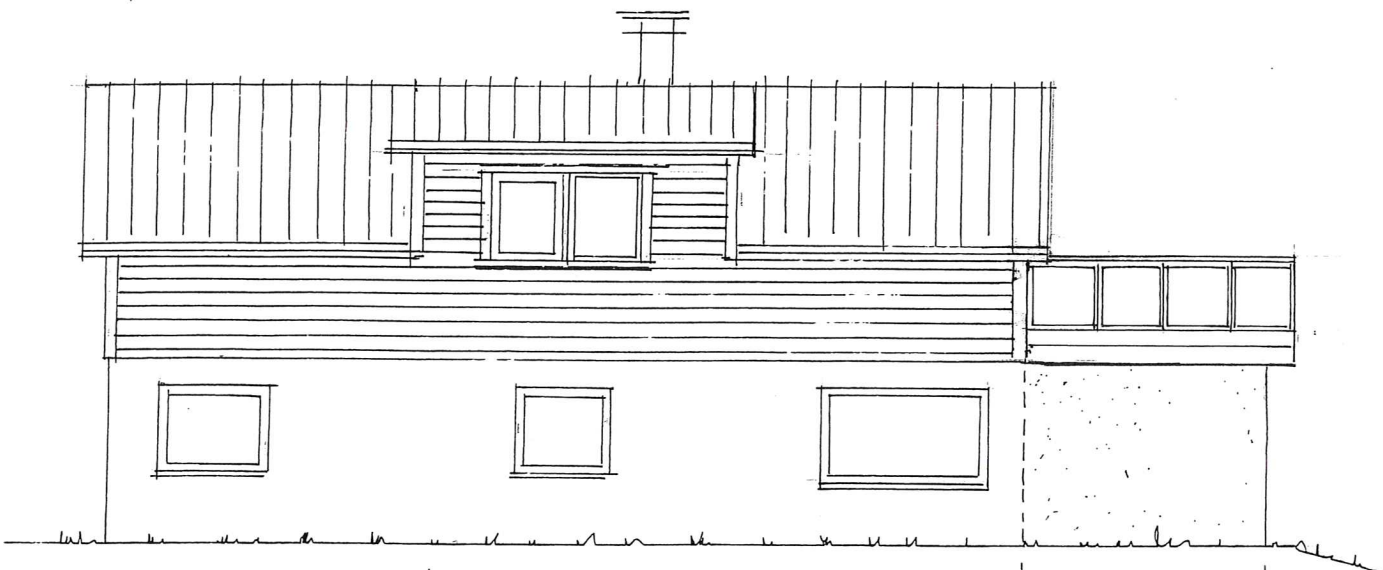
TILBYGG Fasade mot Nord-Øst
