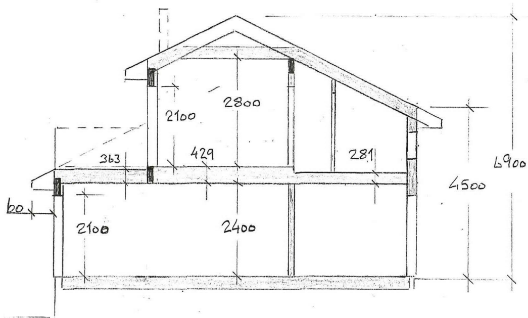
SNITT B-B
