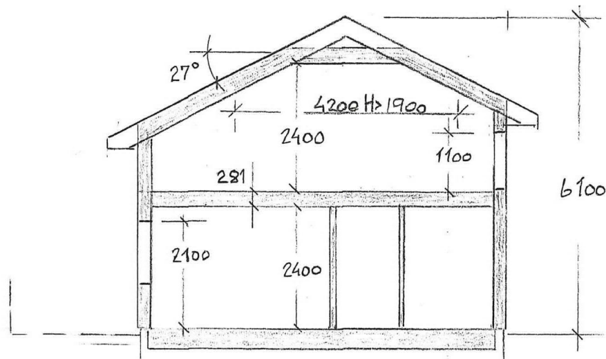
SNITT A-A
