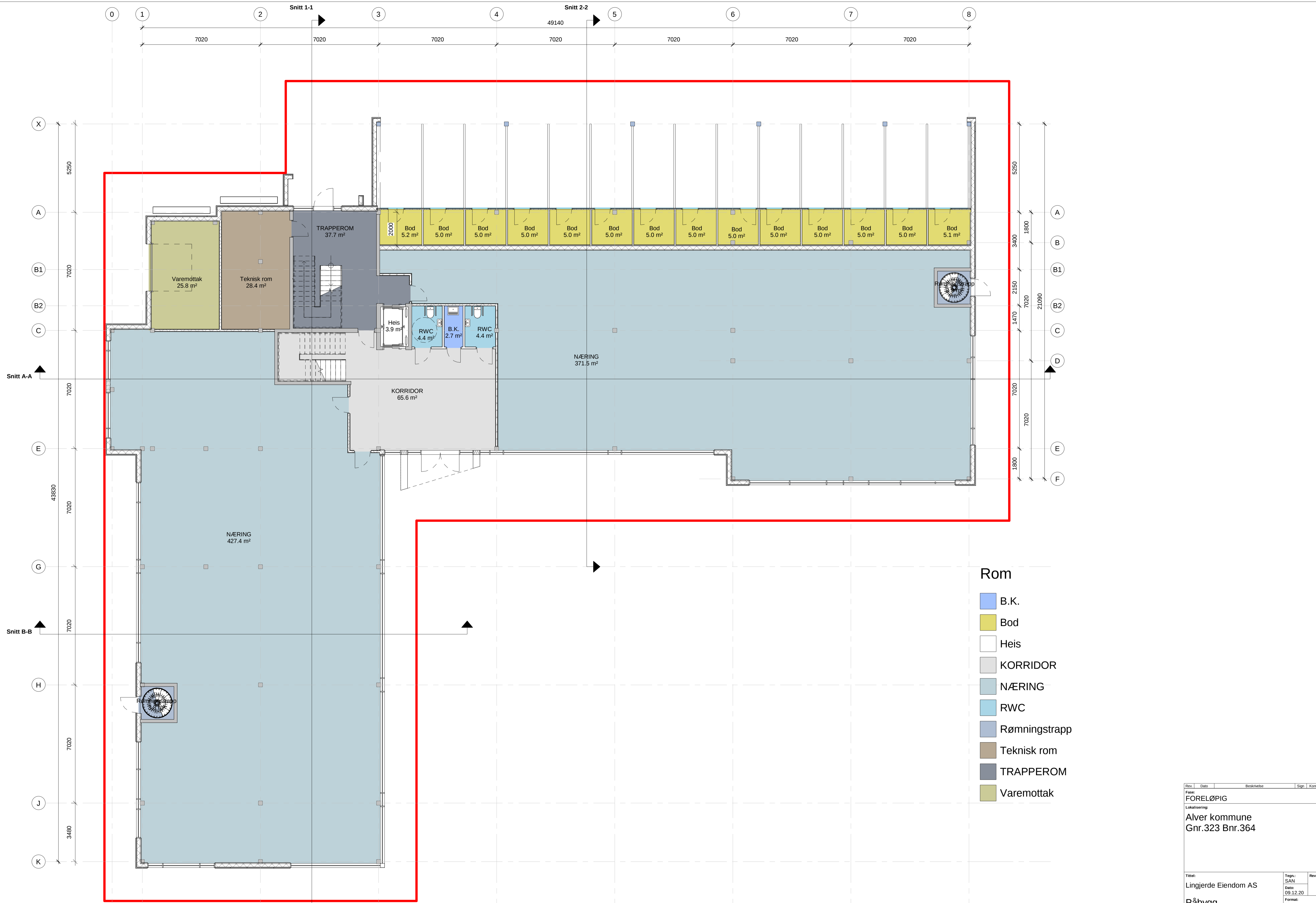
1 Plan 01 1 : 100
