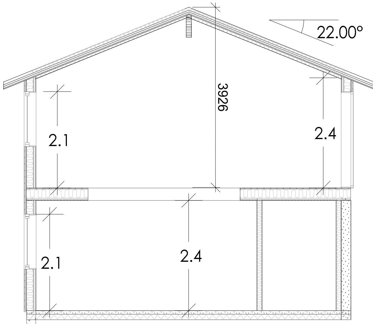
SNITT B-B
