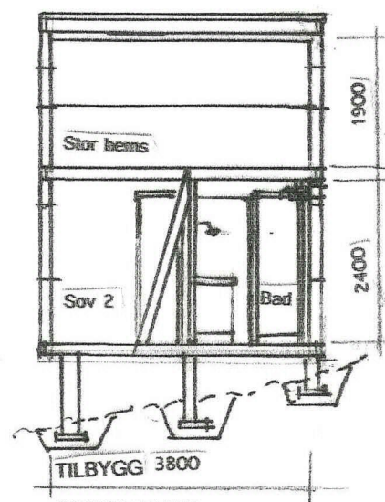
SNITT B-B
