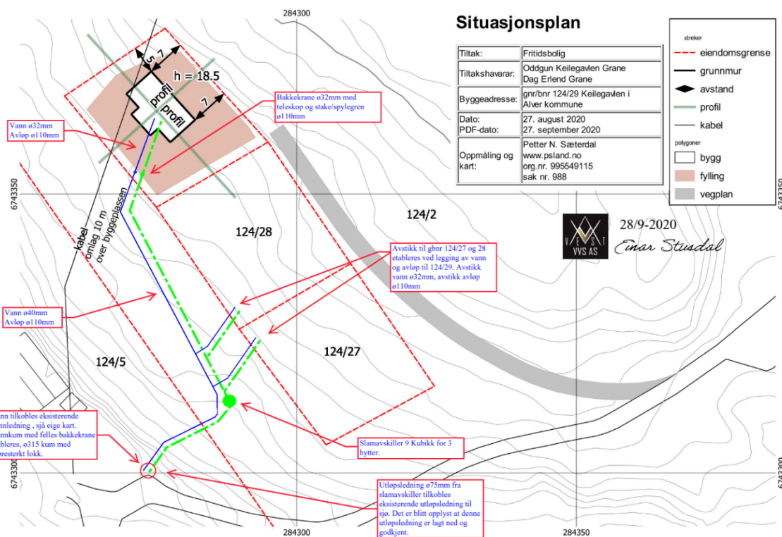
Figur 3. Innsendte situasjonsplan som viser tomter med tilhørende veg og VA
