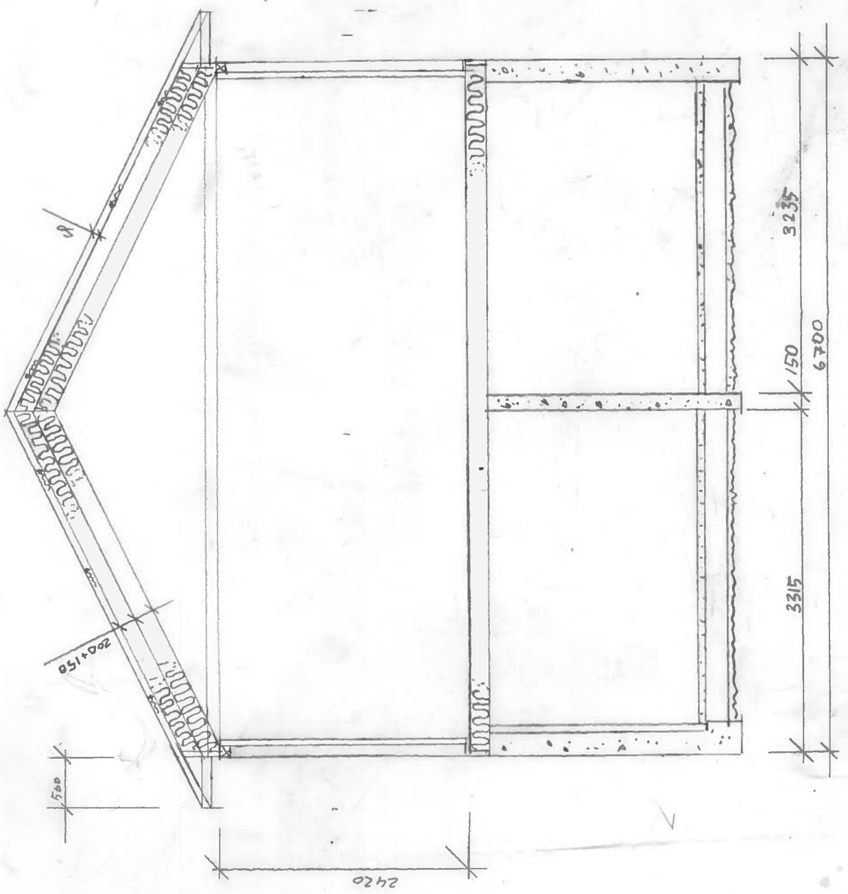
SNITT B-B
