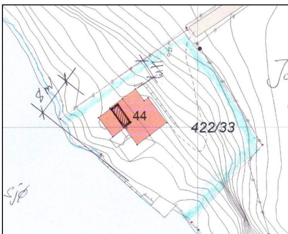
Situasjonsplan
