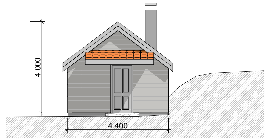
fasade Øst
