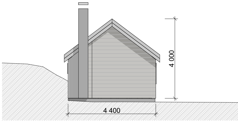
fasade Vest
