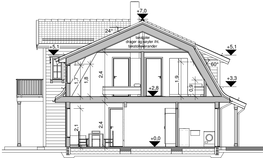
A 1 : 100
