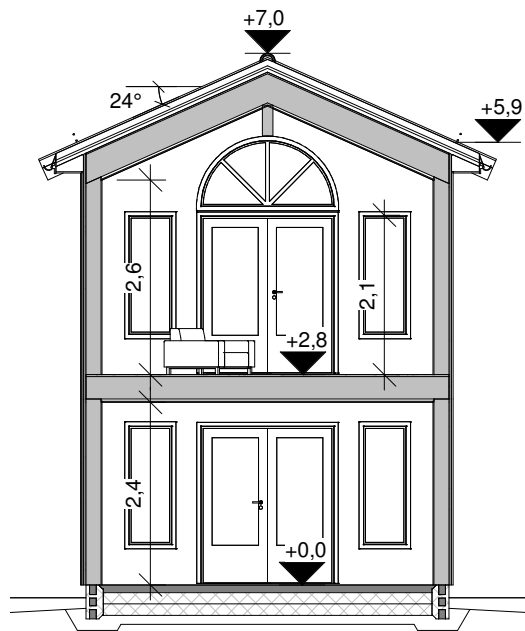
B 1 : 100
