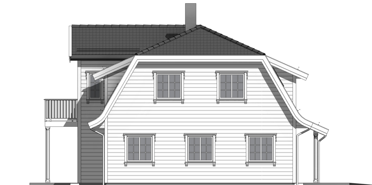
sør 1 : 100
