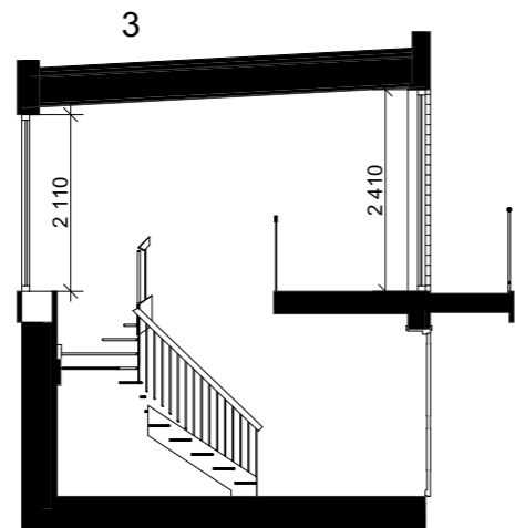
Snitt C
