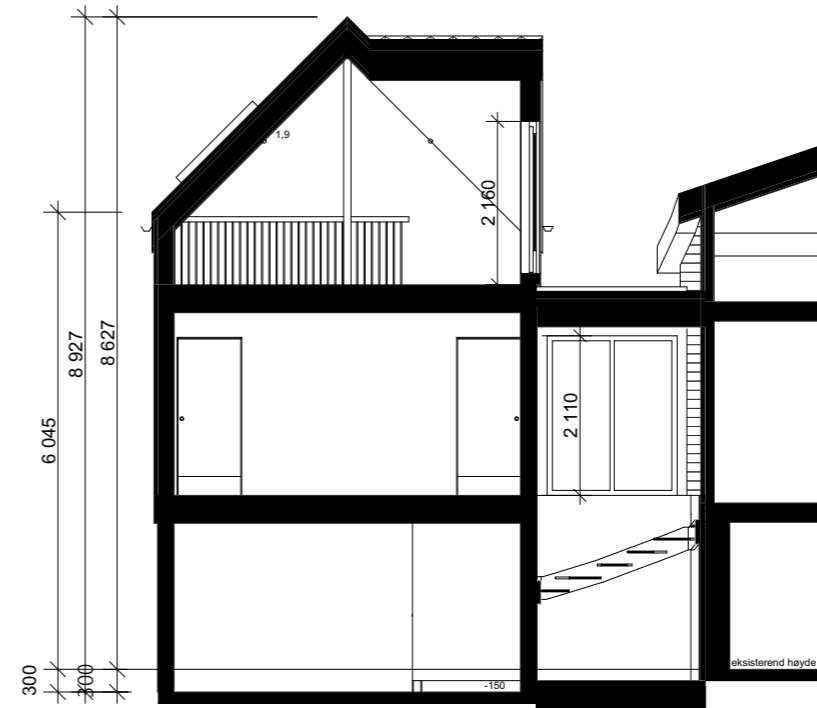
Snitt B
