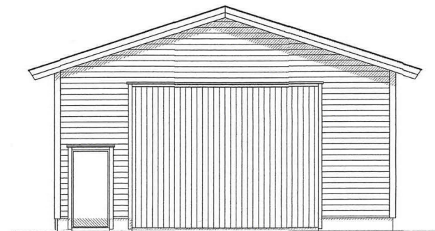
Fasade mot sør
