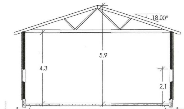
Snitt A-A
