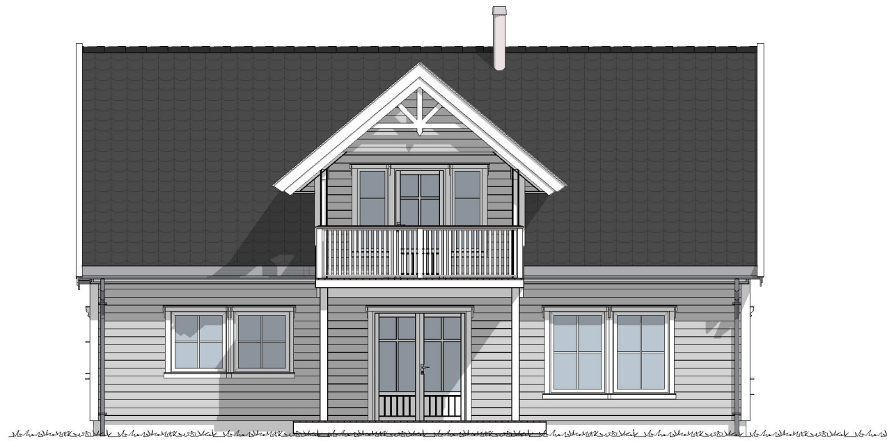
1:100 Fasade 1
