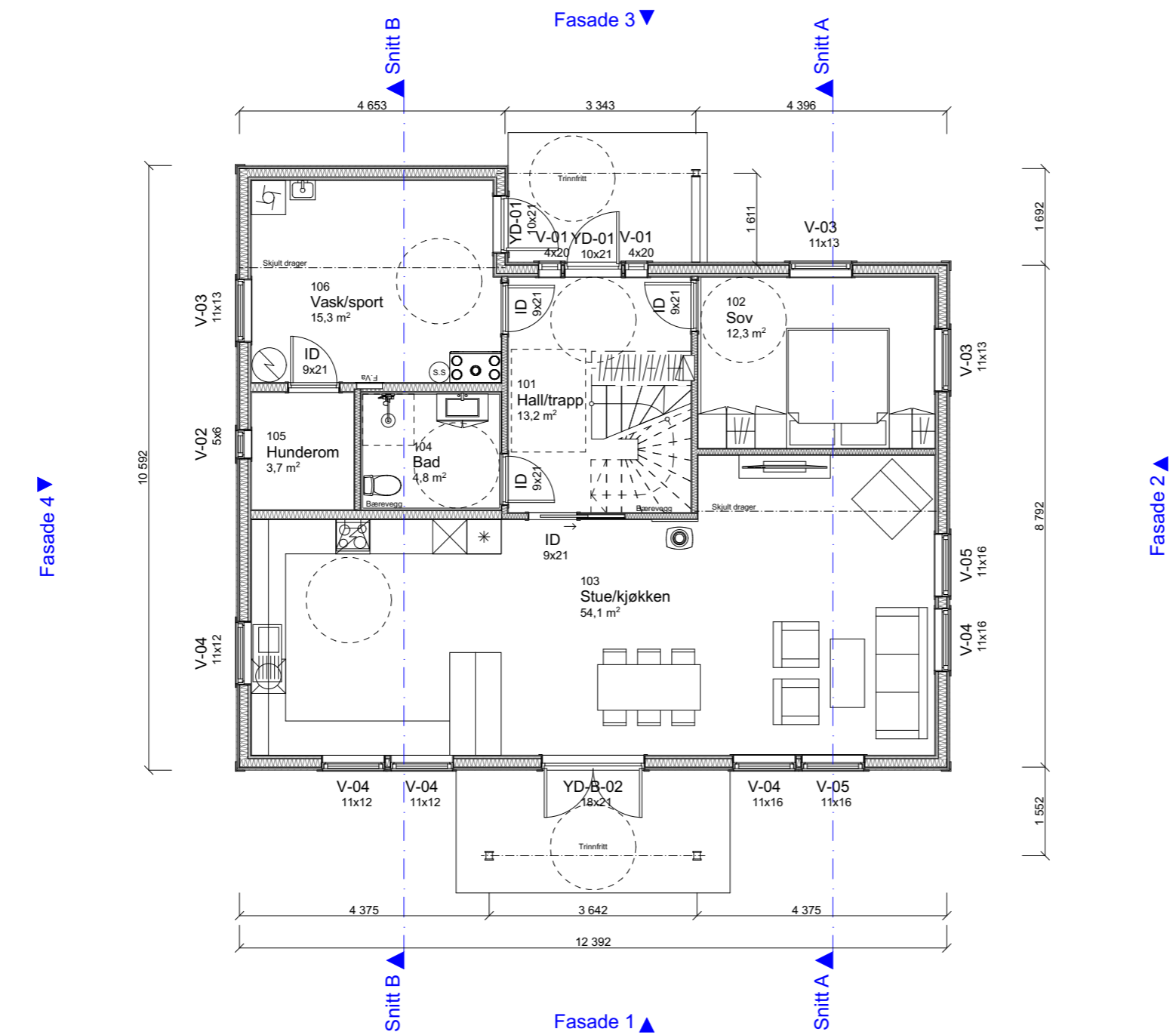
1:100 1. Etasje
