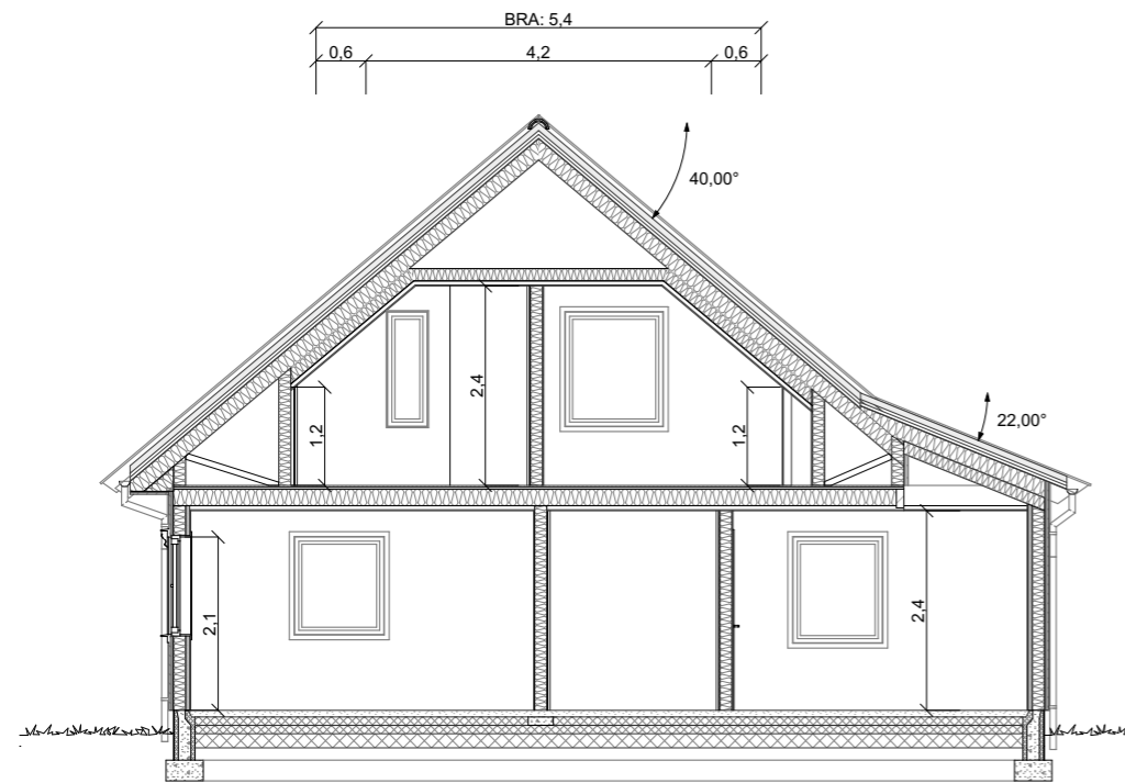
1:100 Snitt B
