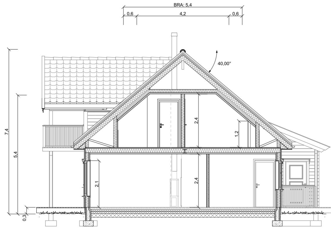
1:100 Snitt A
