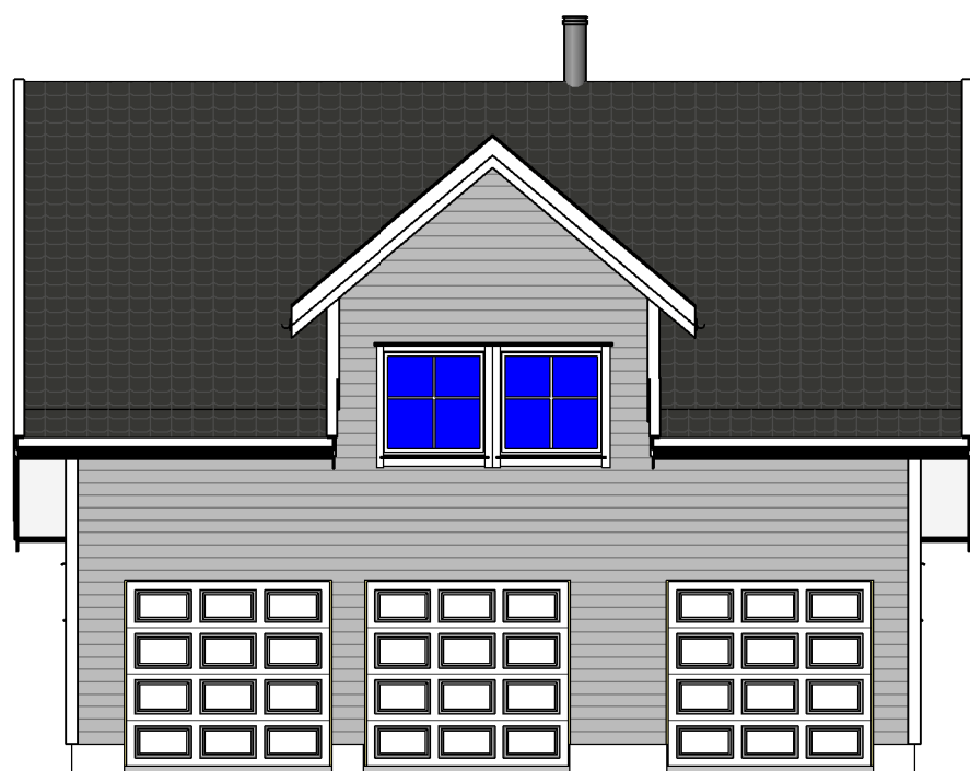
FASADE 1 1 : 100
