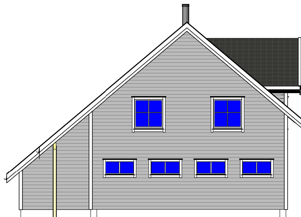
FASADE 4 1 : 100
