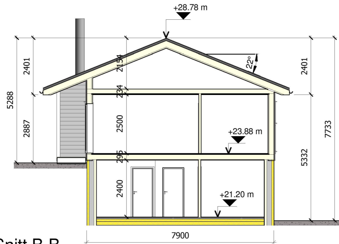
Snitt B-B 1 : 100
