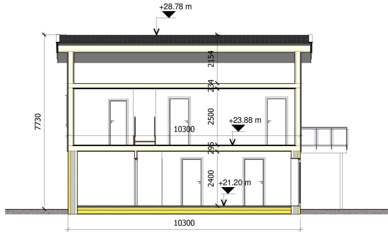
Snitt A-A 1 : 100
