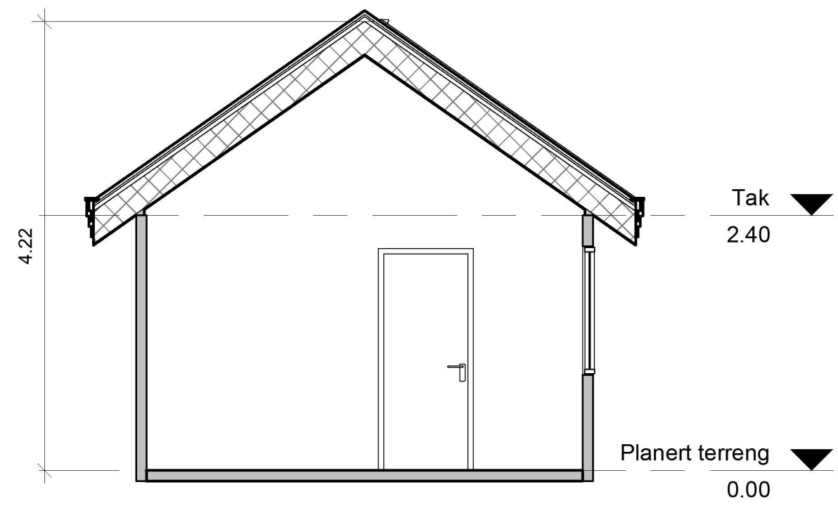
2 Snitt A-A 1 : 50
