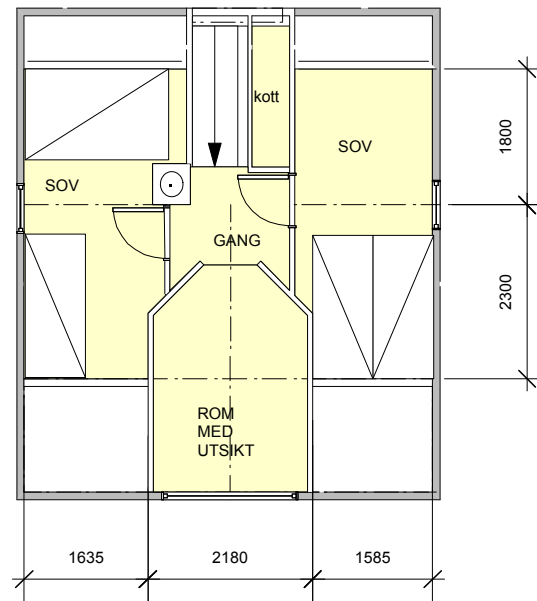
PLAN LOFT
