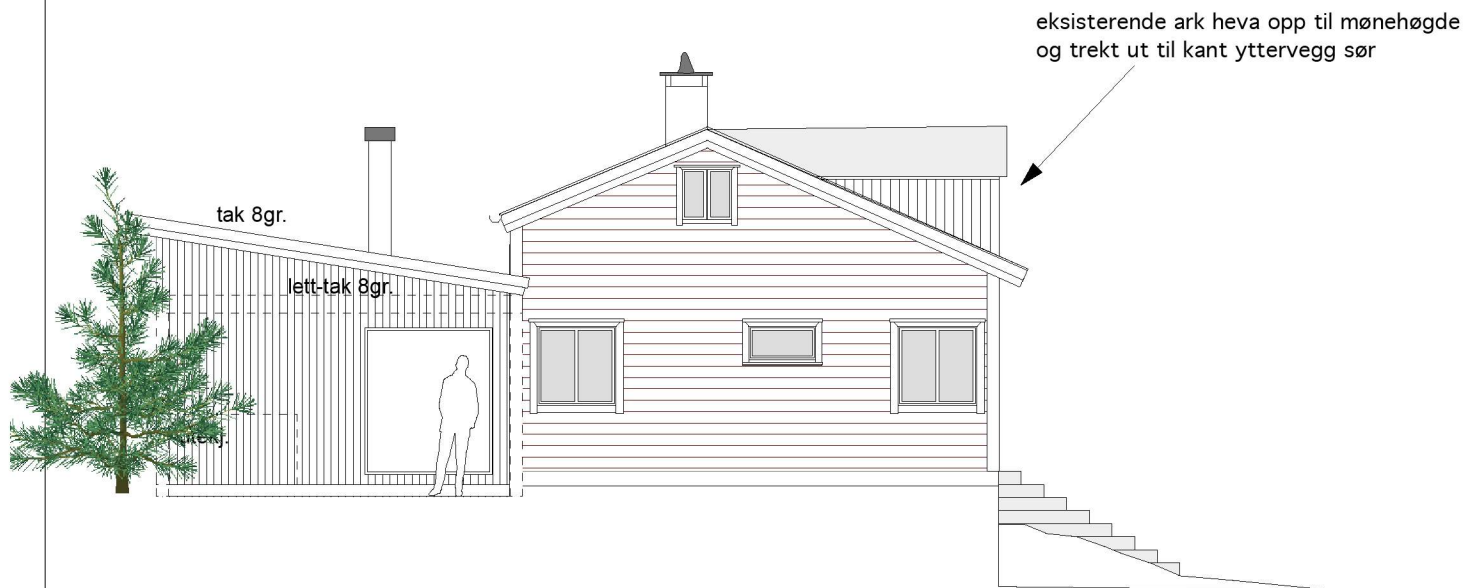
FASADE VEST
