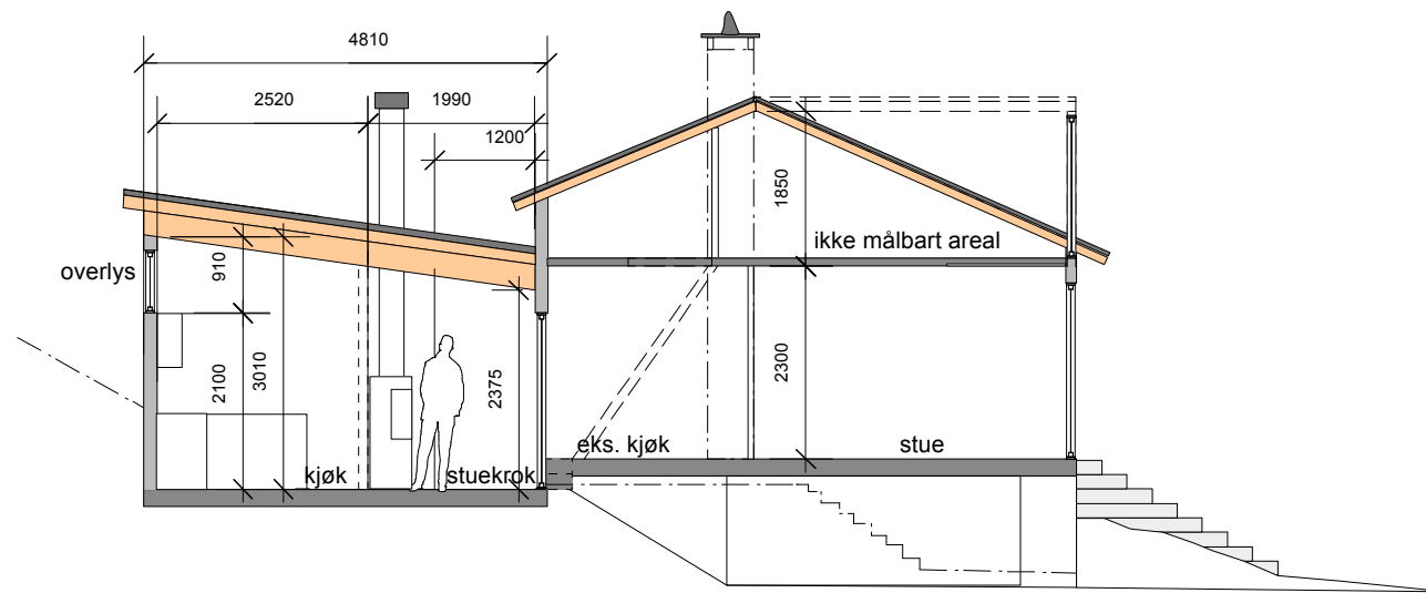
SNITT A
