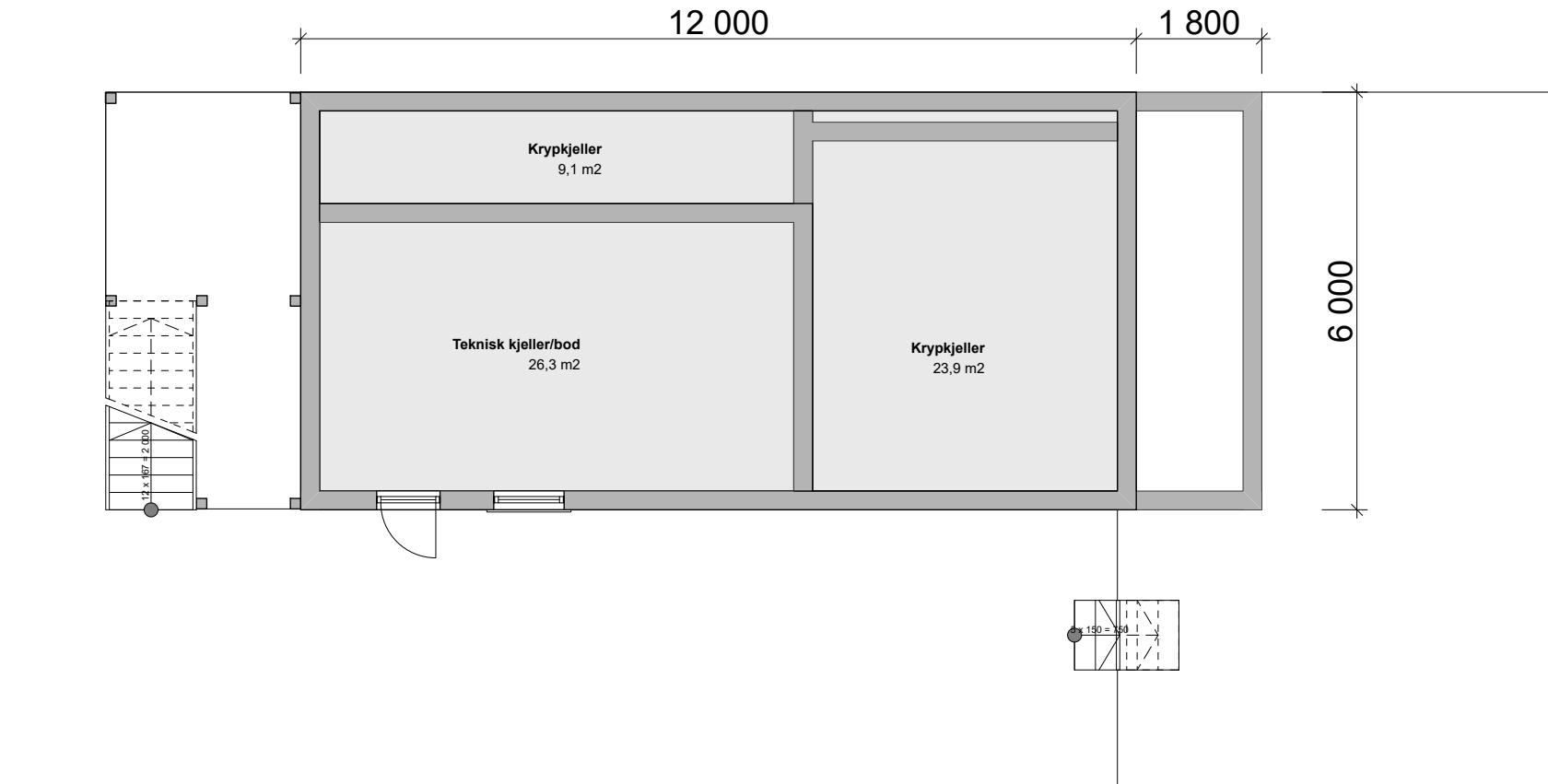
1:100 Kjellarplan
