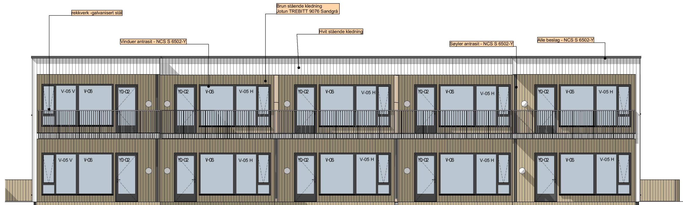
Fasade Vest
