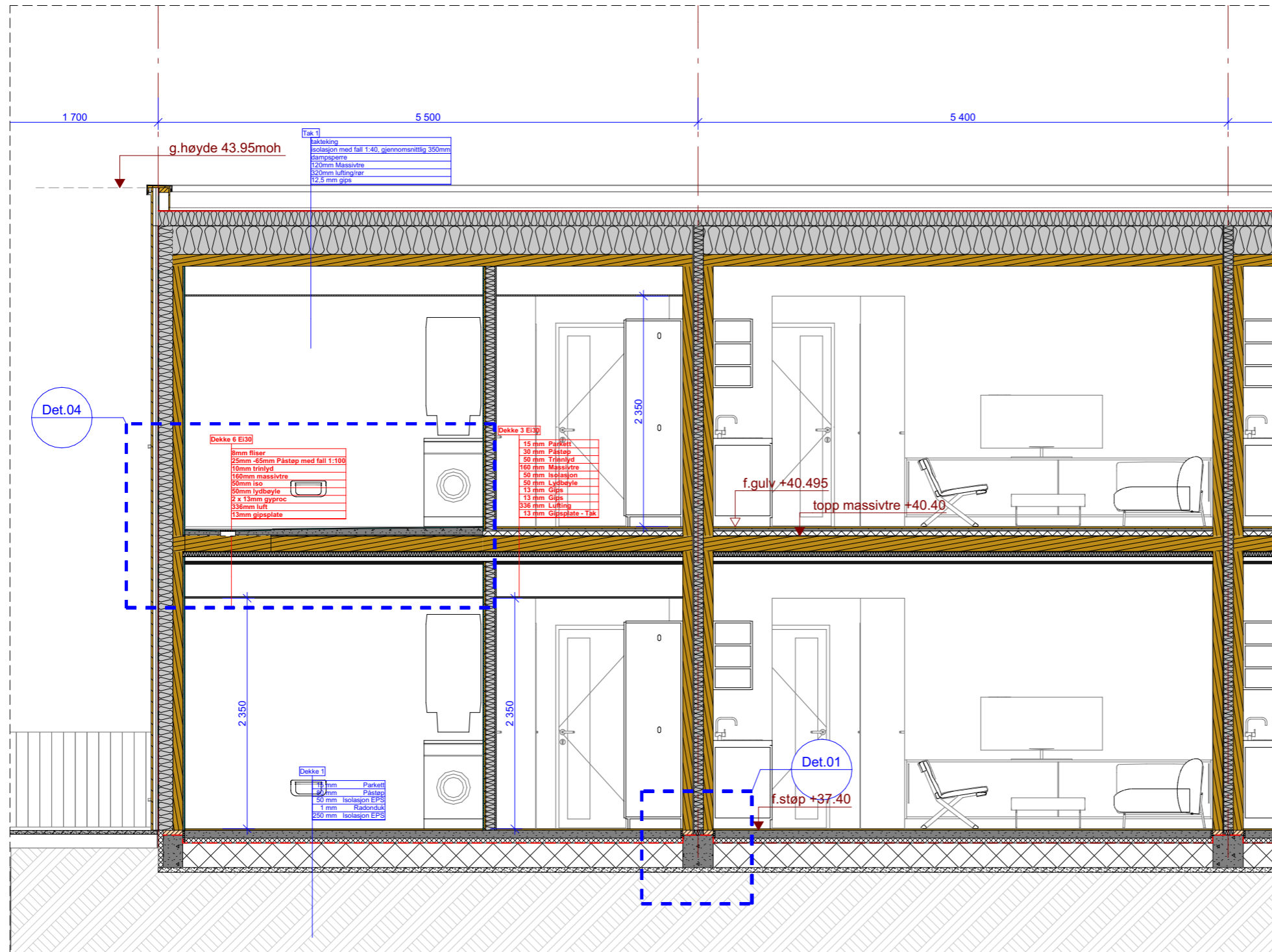
Snitt C
