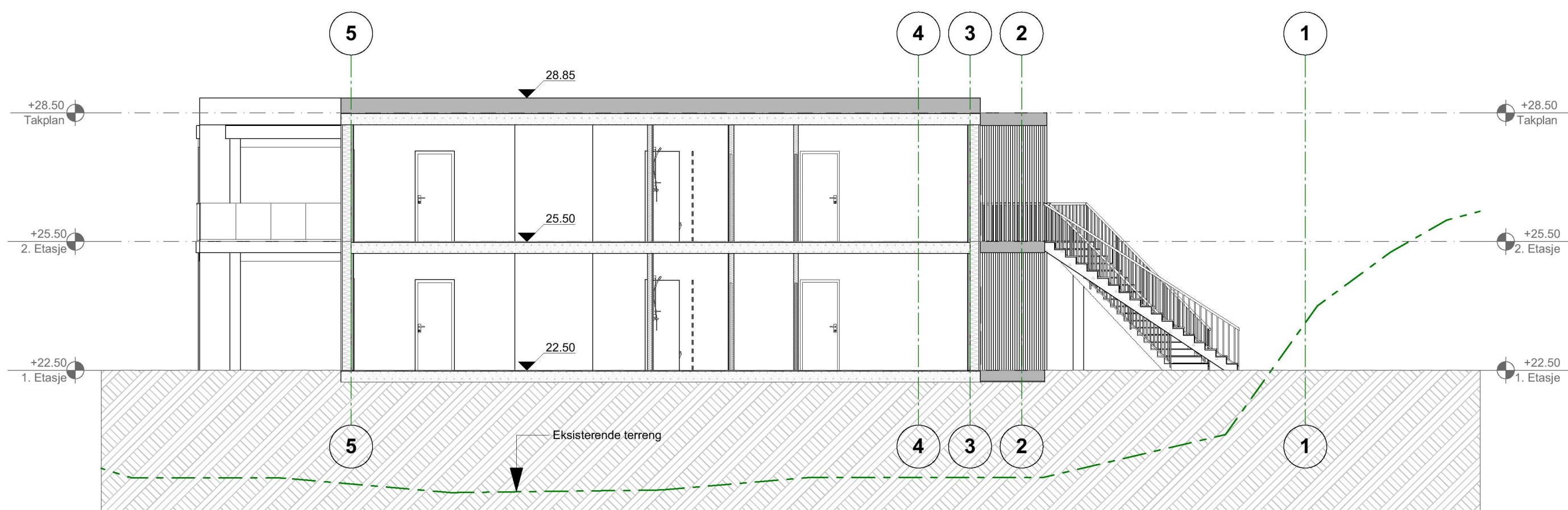
Snitt BB
