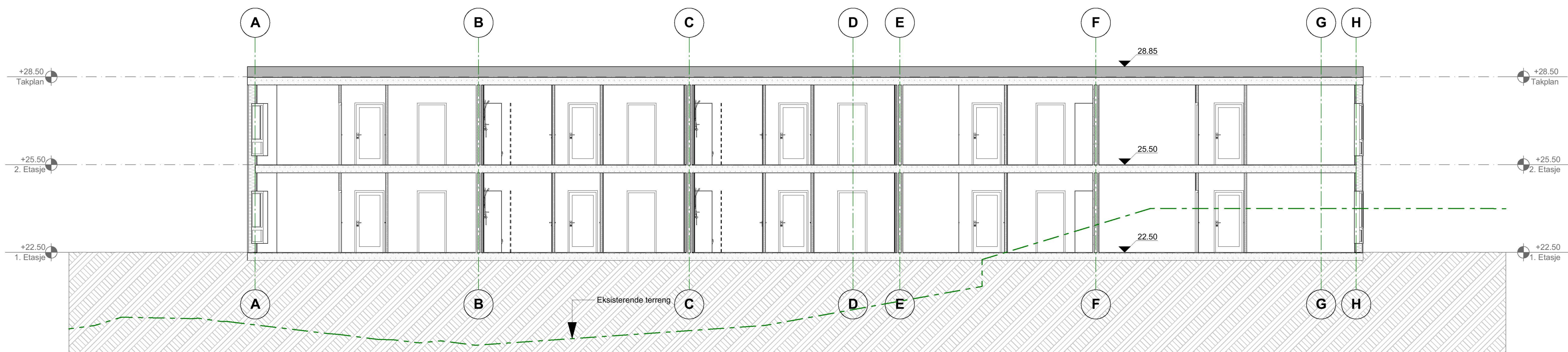
Snitt AA
