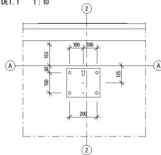
DET. 1 1 : 10
