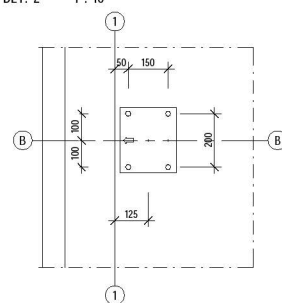
DET. 2 1 : 10
