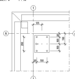
DET. 3 1 : 10
