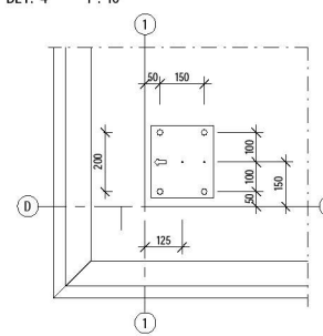
DET. 4 1 : 10
