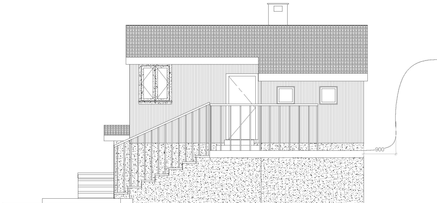
① Fasade mot nordøst 1 : 20
