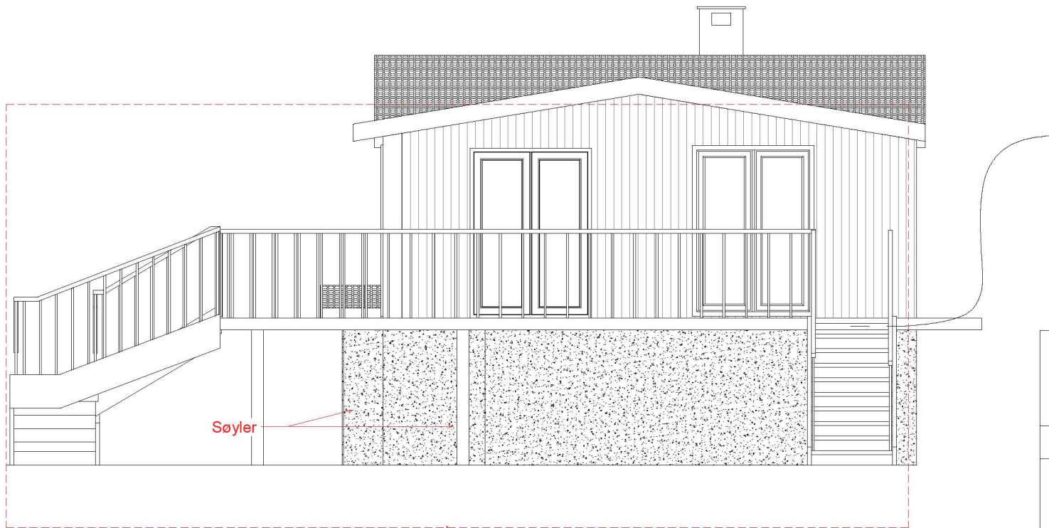
① Fasade mot nordøst 1 : 20
