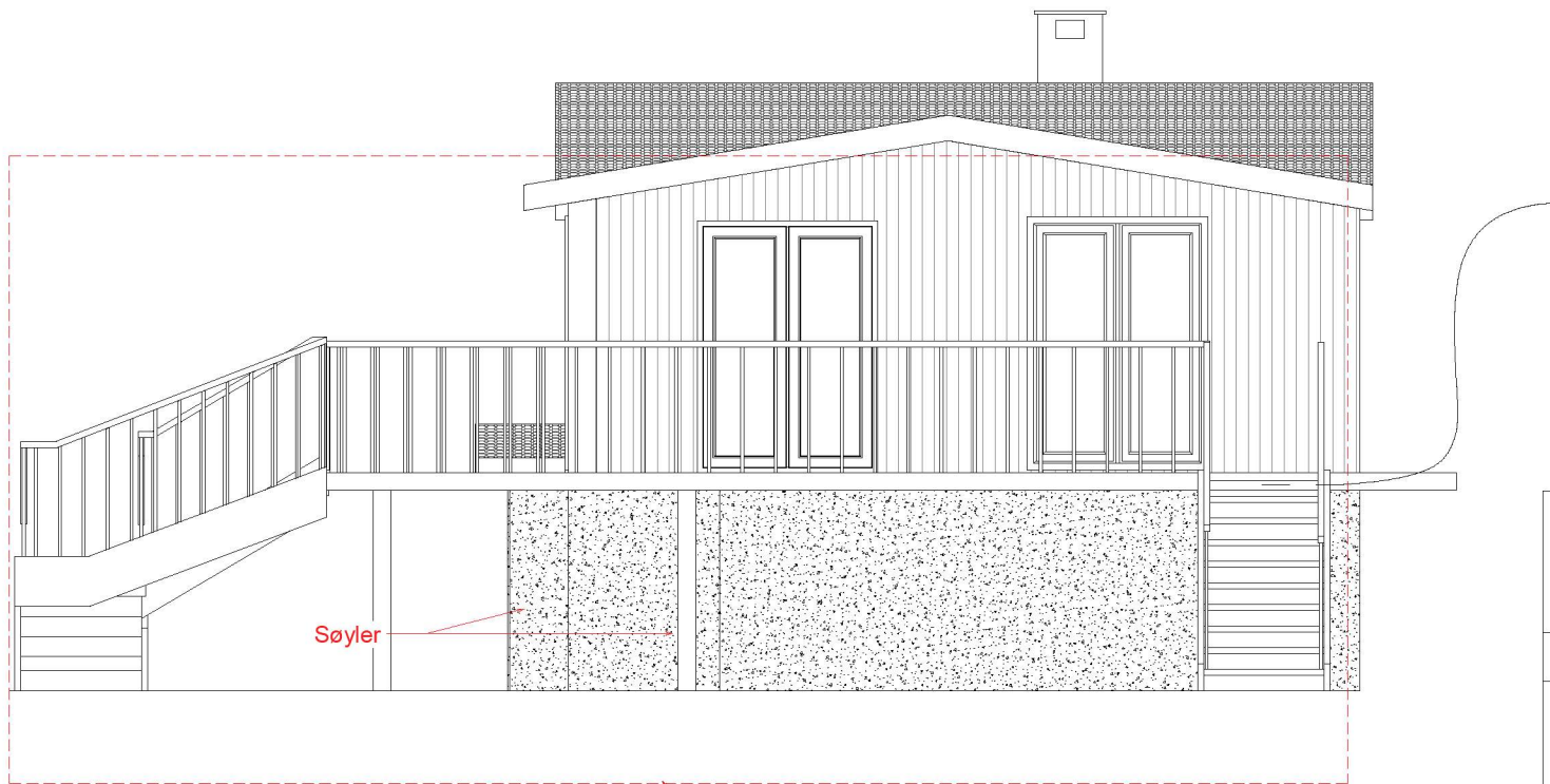
1 Fasade mot nordøst 1 : 20
