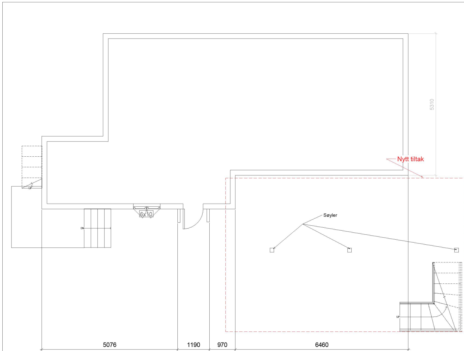
1 Plan U-etasje 1 : 25
